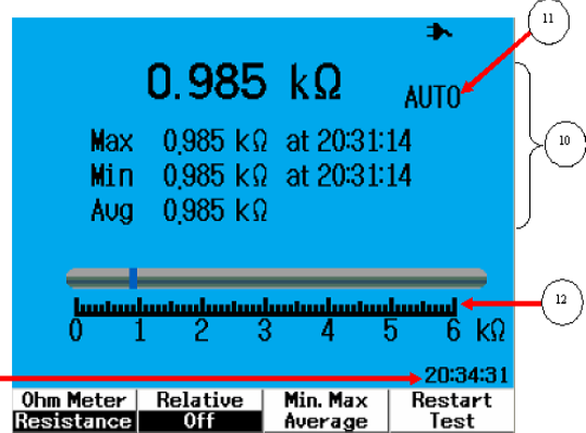
圖 2 電表顯示器
